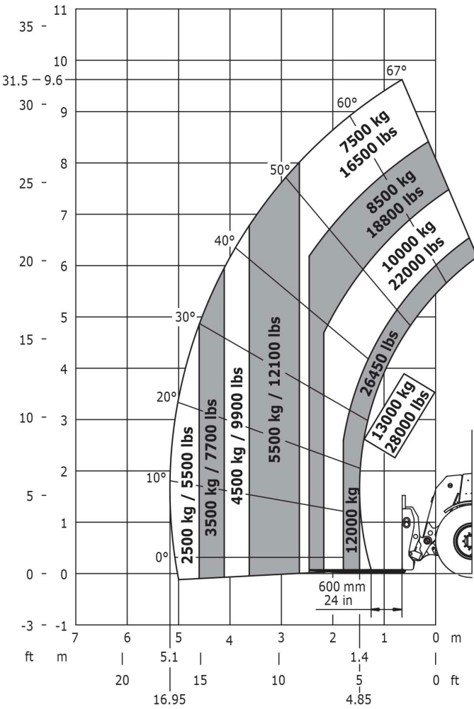
Maschine auf Rädern mit Gabeln - Lastschwerpunkt 600 mm
