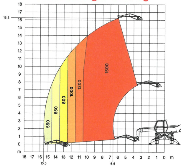
Geschwenkt auf Stützen mit Kranausleger 1500 kg
