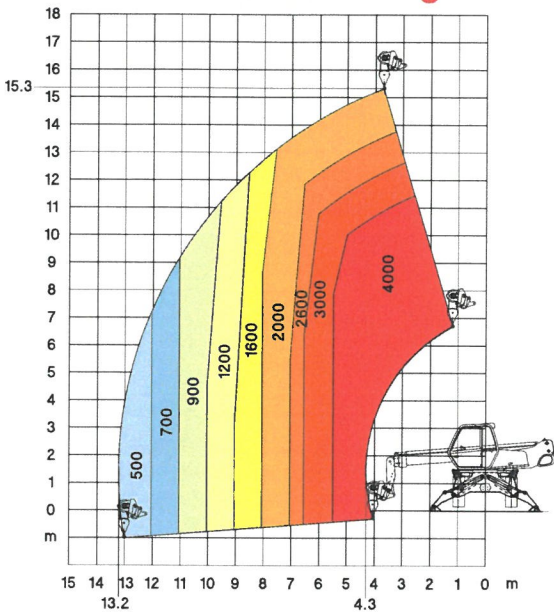
Geschwenkt auf Stützen mit Seilwinde 4000 kg
