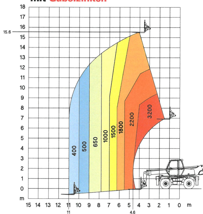
Frontal auf Rädern mit Gabelzinken
