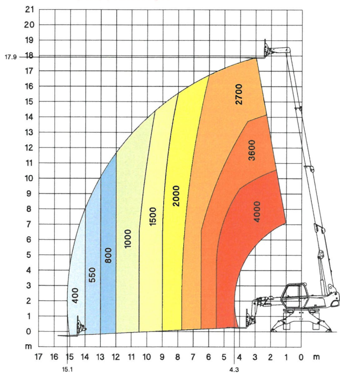
Geschwenkt auf Stützen mit Gabelzinken
