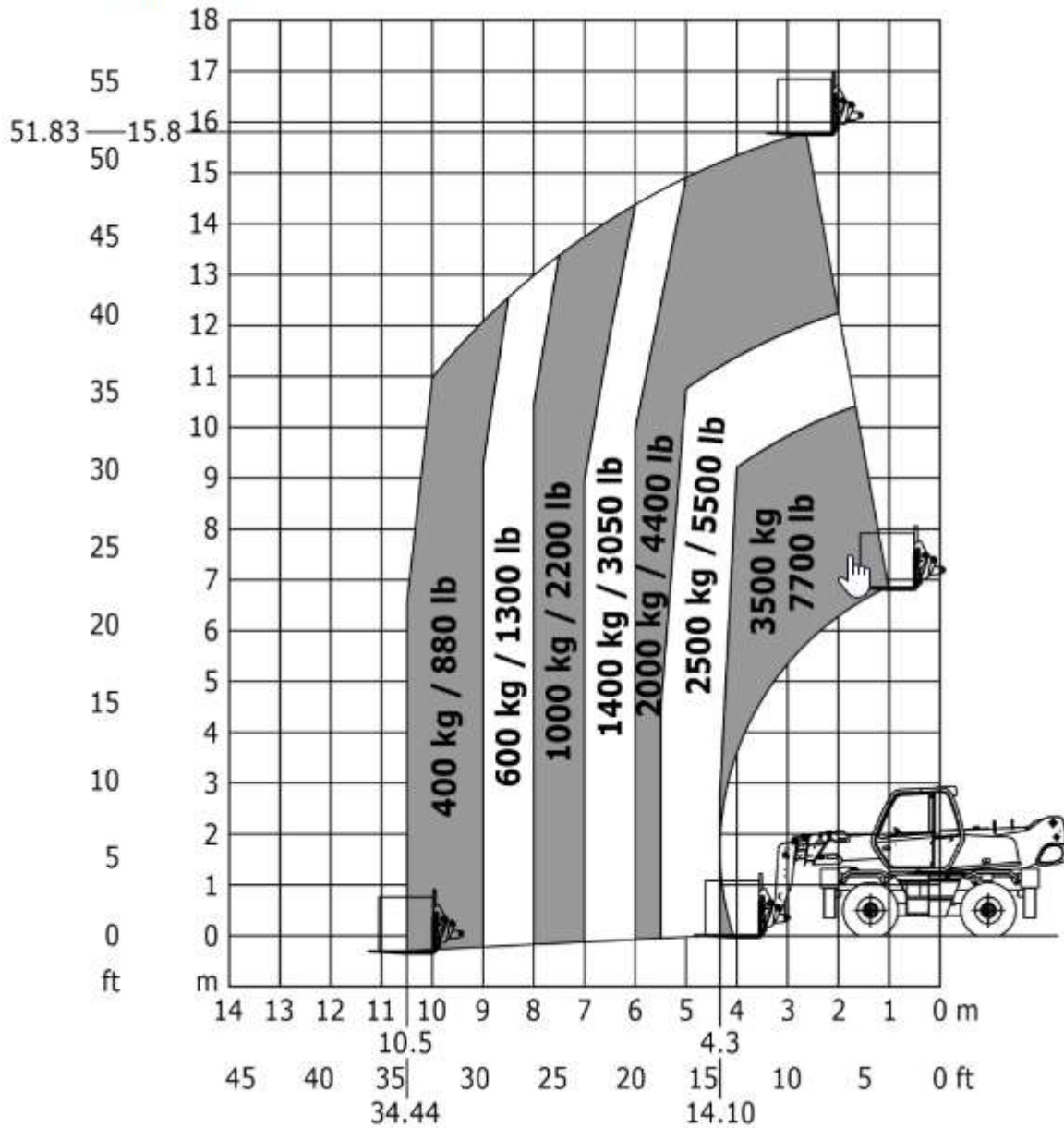
Lastdiagramm (EN1459-B) :
