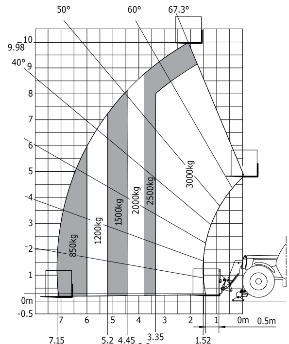
Maschine mit Gabeln auf Stützen CDG 500 mm
