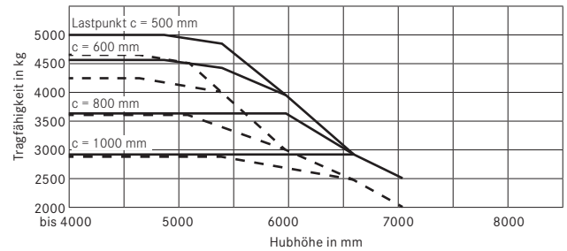
Tragfähigkeiten RX 60-50 Dreifach-Hubgerüst/Zwillingbereifung
