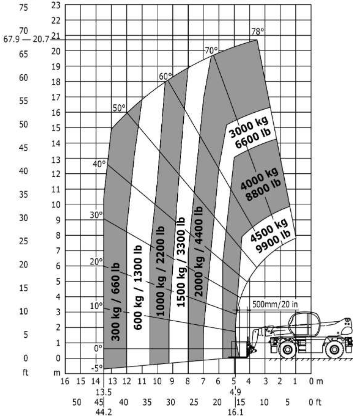
Lastdiagramm (EN1459-B) :
