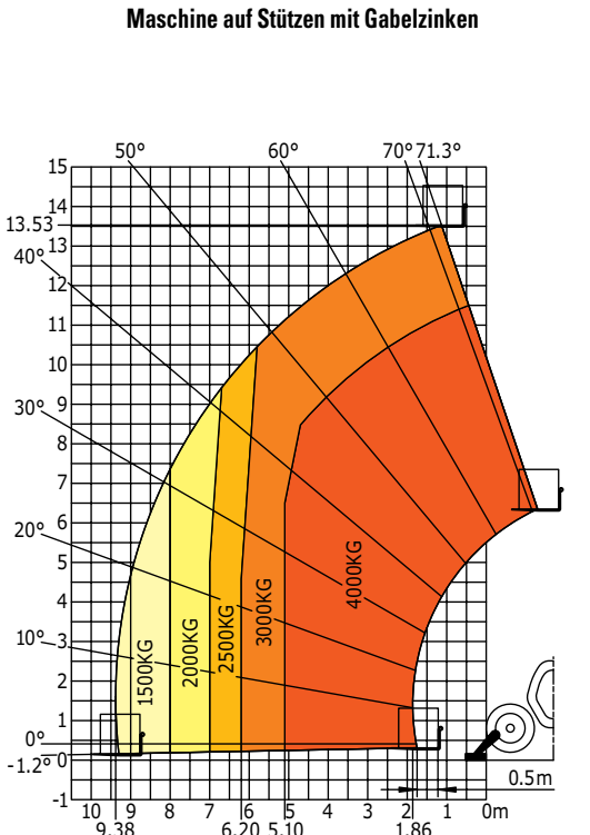
Lastdiagramm Prüfverfahren EN 1459 Zusatz B
