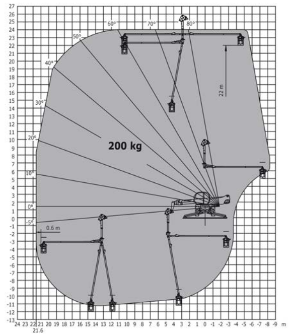
Drehung mit abgesenkten Stützen mit 3D negativ
