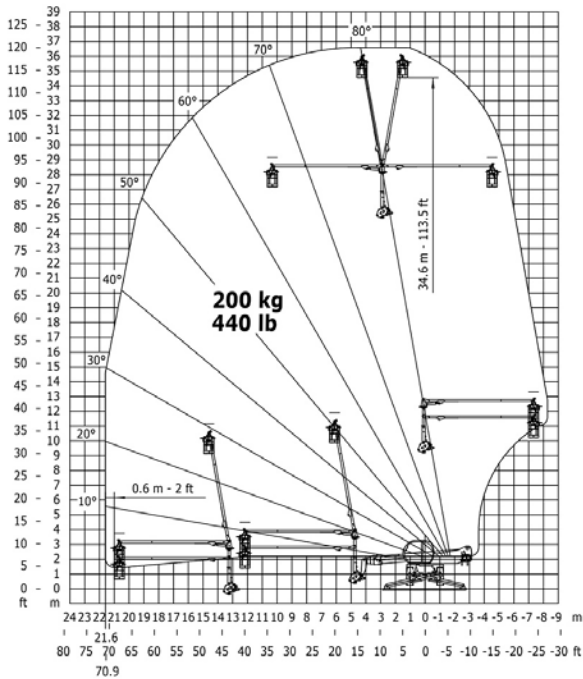
Drehung mit abgesenkten Stützen mit 3D positiv / negativ
