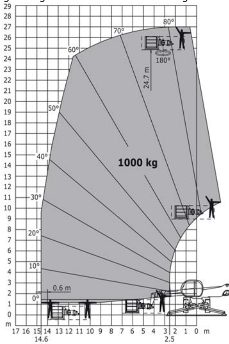
Drehung an abgesenkten Stützen mit 1000 kg Arbeitskorb
