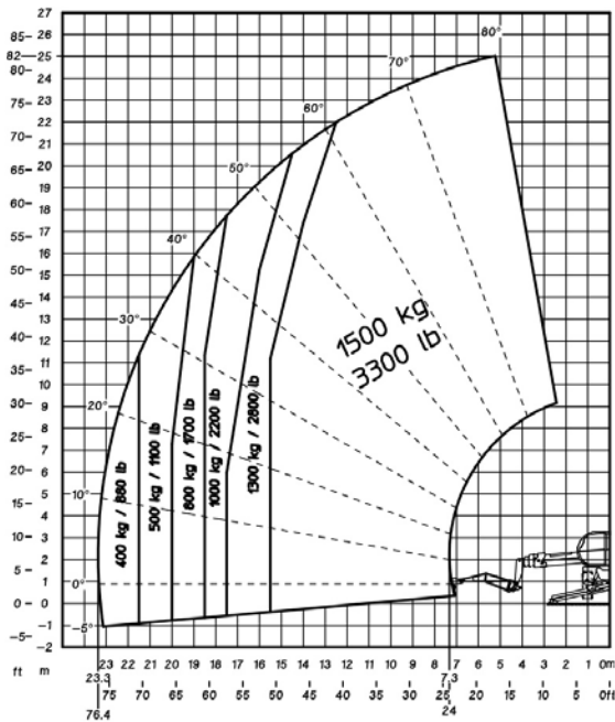
Drehung an abgesenkten Stützen mit 1500 kg Ausleger
