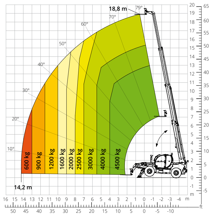
Lastdiagramm mit AUSGEFAHRENEN STÜTZEN ATT-03-042
