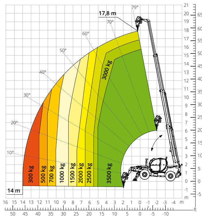
Lastdiagramm mit SEILWINDE 3.500 kg ATT-02-002
