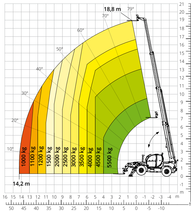
Lastdiagramm mit AUSGEFAHRENEN STÜTZEN ATT-03-040
