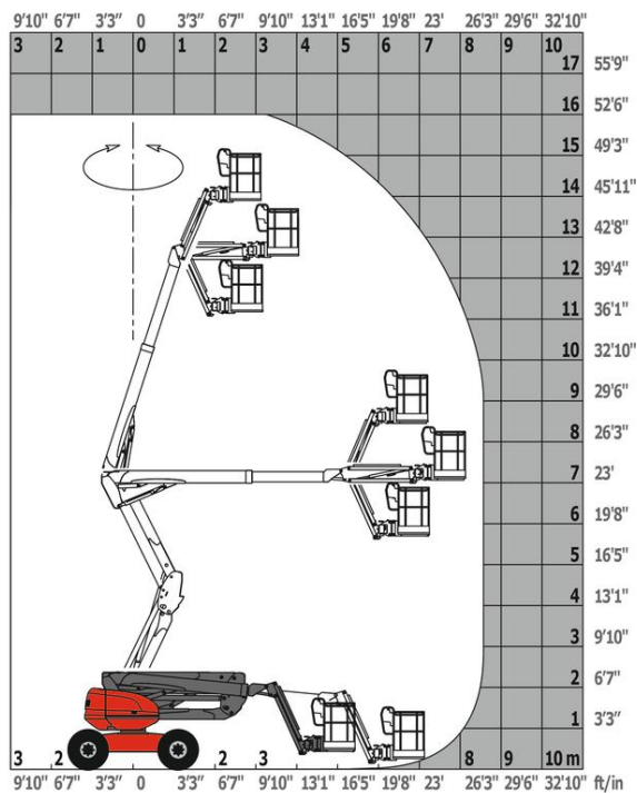
Lastdiagramm für Hubarbeitsbühne
