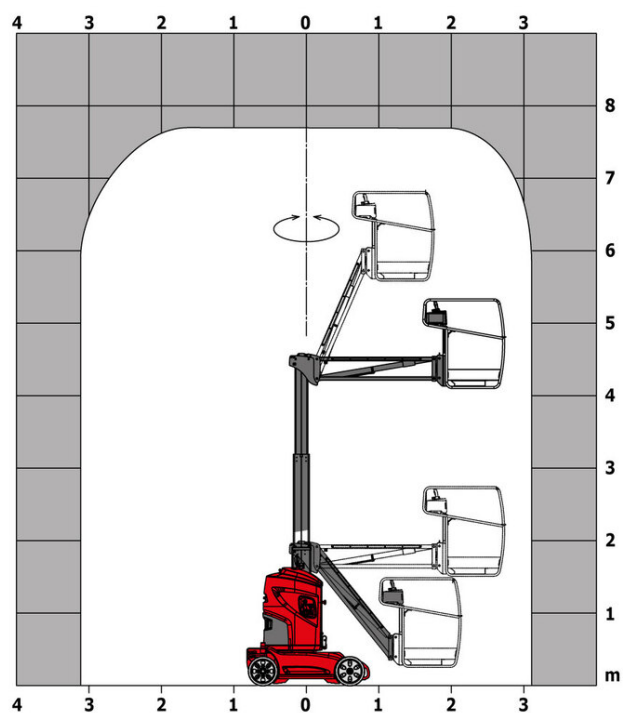
Lastdiagramm
