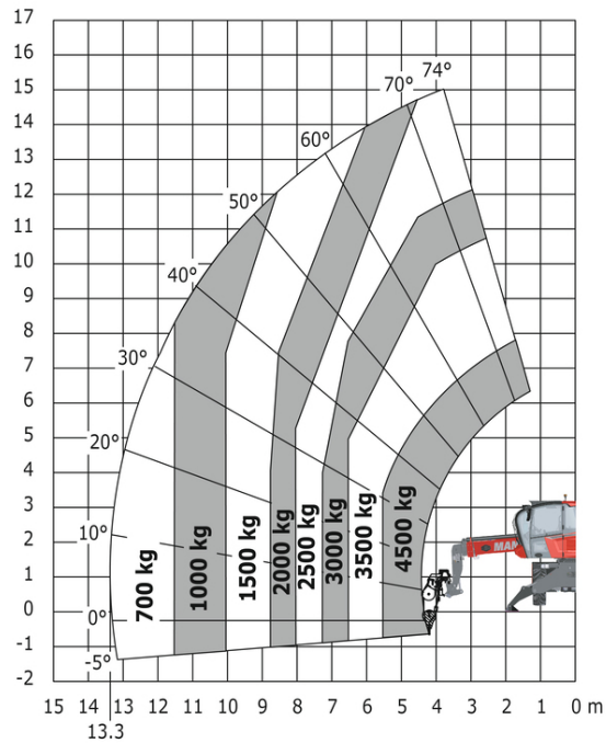
Drehung mit abgesenkten Stützen mit Seilwinde 5000 kg
