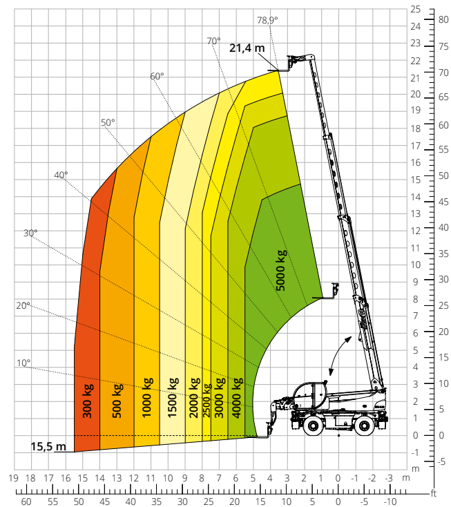
Lastdiagramm FRONTAL AUF REIFEN ATT-03-004
